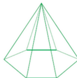
Pyramide à base hexagonale
