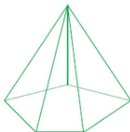
Pyramide à base pentagonale
